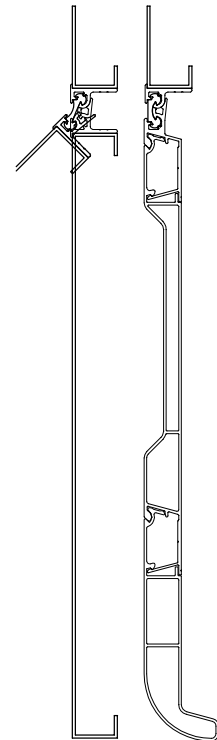
455 811 1940 gr / m 7.2 m anod
