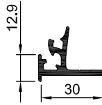
270 026 500 gr / m 5.0 m anod
